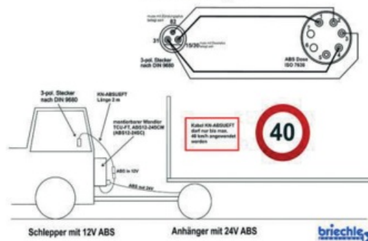
Nachrüst-Design für Anhänger ABS24V mit 12 V Schlepper
